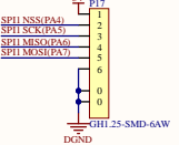
SPI接口
