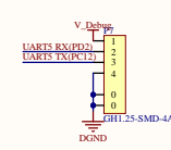
UART5调试接口
