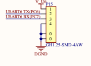
USART6裁判系统接口
