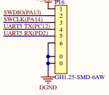
联合调试接口
