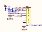
SWD调试接口
