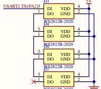
WS2812显示
