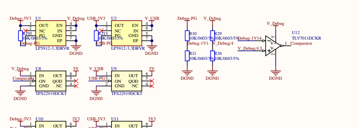
调试&USB输入保护
