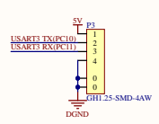
USART3板级通信接口
